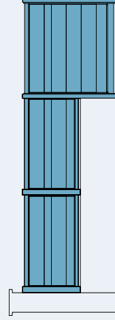
Modèle ÉLYSIUM 1 Avec lames larges horizontales 250 x 25 mm et lames Led 125 x 25 mm (sans Led)
