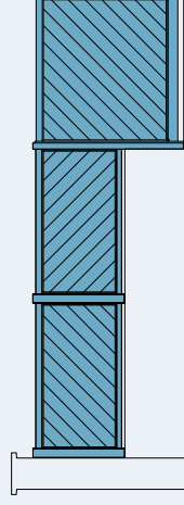
Modèle JABAL Avec lames 125 x 25 mm inclinées à 45° (option)
