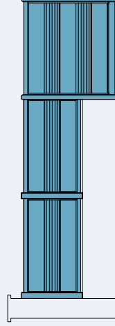
Brise-vue ELBE 2 (avec clôture sur muret ELBE 1) La clôture ELBE 2 est disponible à partir de H = 1,26 m Modèles avec lames à effet bardage 250 x 25 mm et lames larges
