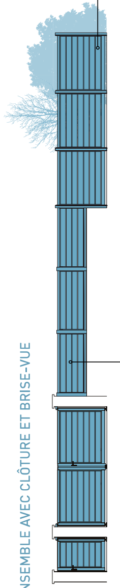
Brise-vue BORNÉO Brise-vue en pente réalisable (pente 10% maxi) Hauteur de brise-vue de 1,50 m à 2 m Entraxe poteaux maxi : 2 m (H ≤ 1,75 m) ou 1,60 m (H > 1,75 m)
