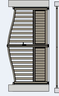
Pose entre piliers (pose en tableau) Ouverture à 90°
