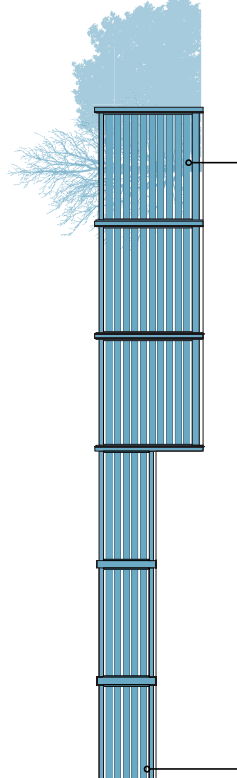
Clôture AVÉA Clôture en pente réalisable (pente 10% maxi) Hauteur de clôture jusqu'à 1,50 m Entraxe poteaux maxi : 2,50 m
