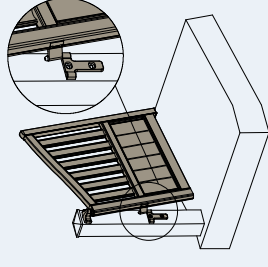
Ouverture avec remonte-pente Pente 5 à 15% selon hauteur du portail Pose en applique : non réalisable
