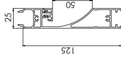
Vue en coupe de la lame intégrant les Leds
