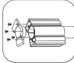
Poteau d'angle éléments orientables
