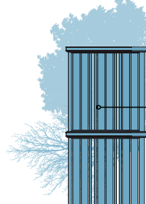
Brise-vue CHYPRE Brise-vue en pente réalisable (pente 10% maxi) Hauteur de brise-vue de 1,50 m à 2 m Entraxe poteaux maxi : 2 m (H ≤ 1,75 m) ou 1,60 m (H > 1,75 m)
