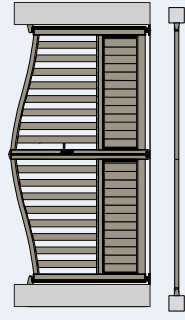
Pose entre piliers (pose en tableau) Ouverture à 90°
