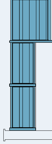
Modèle ÉLYSIUM 2 (disponible à partir de H = 1,01 m) Avec lames larges horizontales 250 x 25 mm et lames Led 125 x 25 mm (sans Led)
